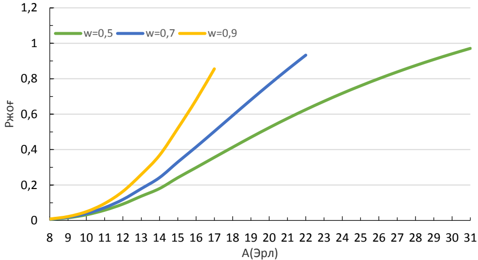
4–сурет – Екінші типтегі шақырулардың жоғалу ықтималдығының келіп түскен жүктемеге тәуелділігі ( V=16 кезінде)
