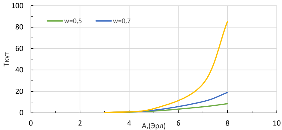
2 – сурет – Бірінші типтегі шақырулардың орташа күту уақытының келіп түскен жүктемеге тәуелділігі (V=8 кезінде)
