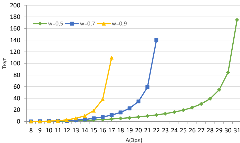
5–сурет – Бірінші типтегі шақырулардың орташа күту уақытының келіп түскен жүктемеге тәуелділігі ( V=16 кезінде)
