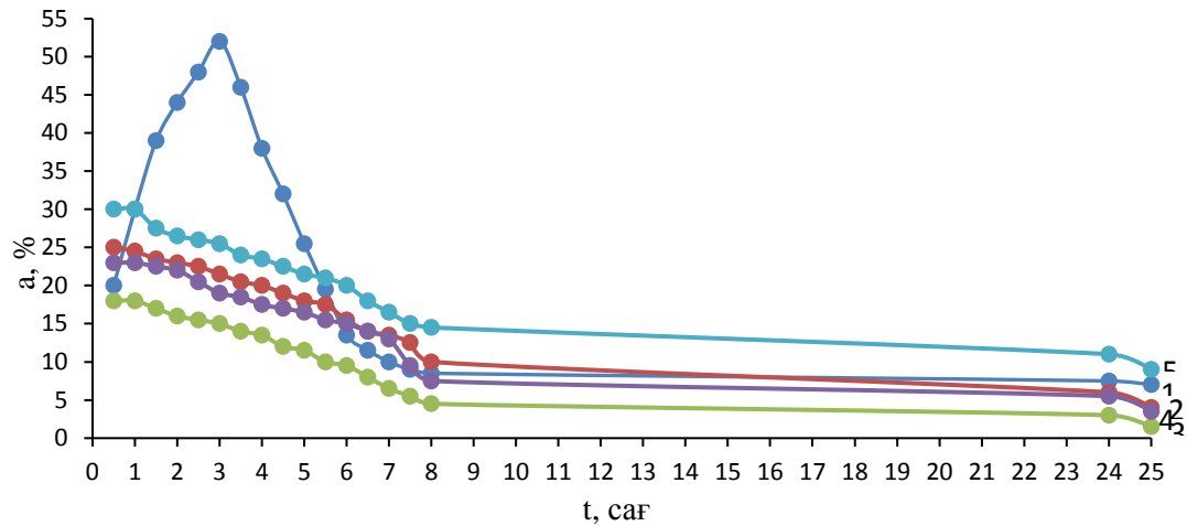
Капсулалардың қалыптасу ортасы: [KCl]=3\text{ M} ; су (1); KCl=3\text{ M} (2); pH=5 (3); 9 (4); 11 (5) . [Геллан]=1\%
