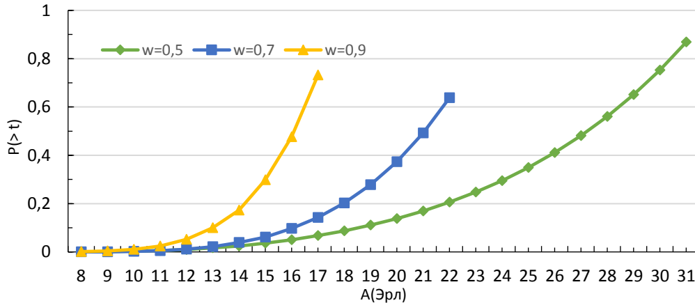
6–сурет – P(>t) ықтималдығының келіп түскен жүктемеге тәуелділігі ( V=16 кезінде)
