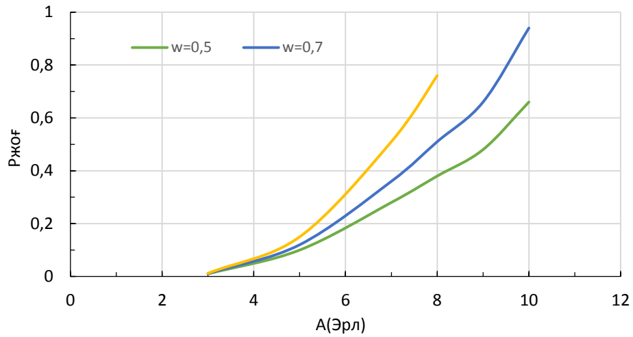
1–сурет – Екінші типтегі шақырулардың жоғалу ықтималдығының келіп түскен жүктемеге тәуелділігі (V=8 кезінде)
