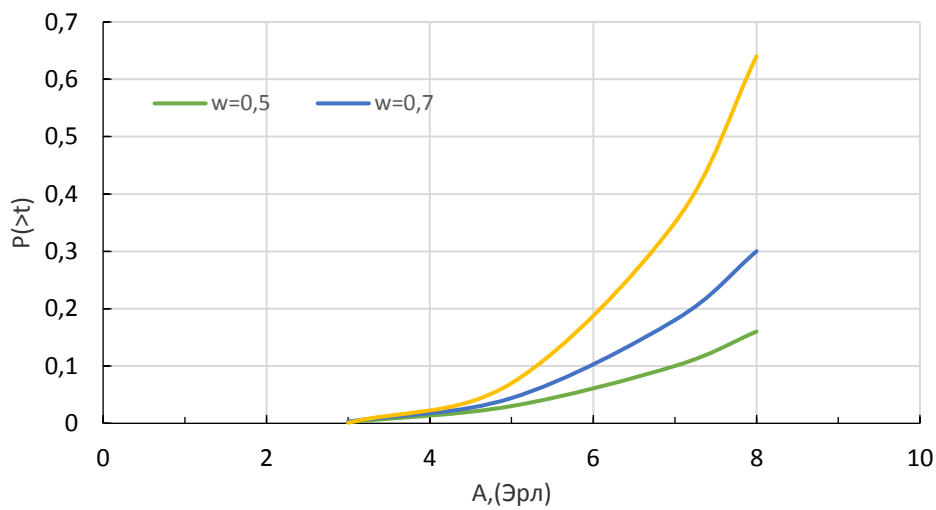
3–сурет – P(>t) ықтималдығының келіп түскен жүктемеге тәуелділігі (V=8 кезінде)
