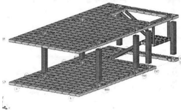
А – расчетная схема блока; Б – фрагмент блока
