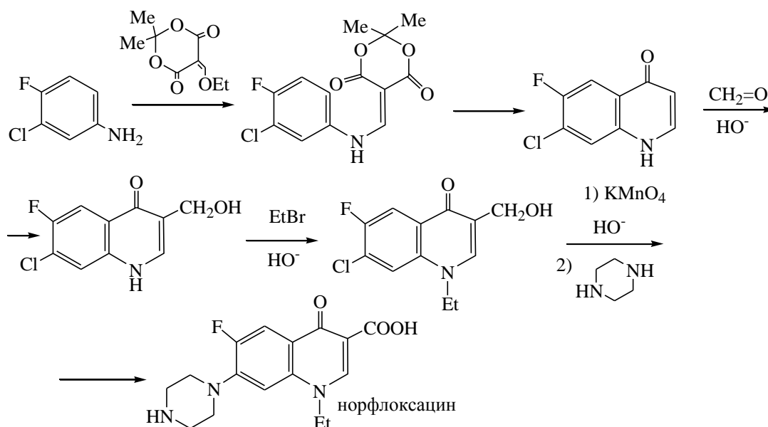
Рисунок 9 – Синтез норфлоксацина
