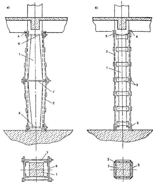
Рисунок 4 – Усиление колонны предварительно напряженной односторонней металлической распоркой [4]
